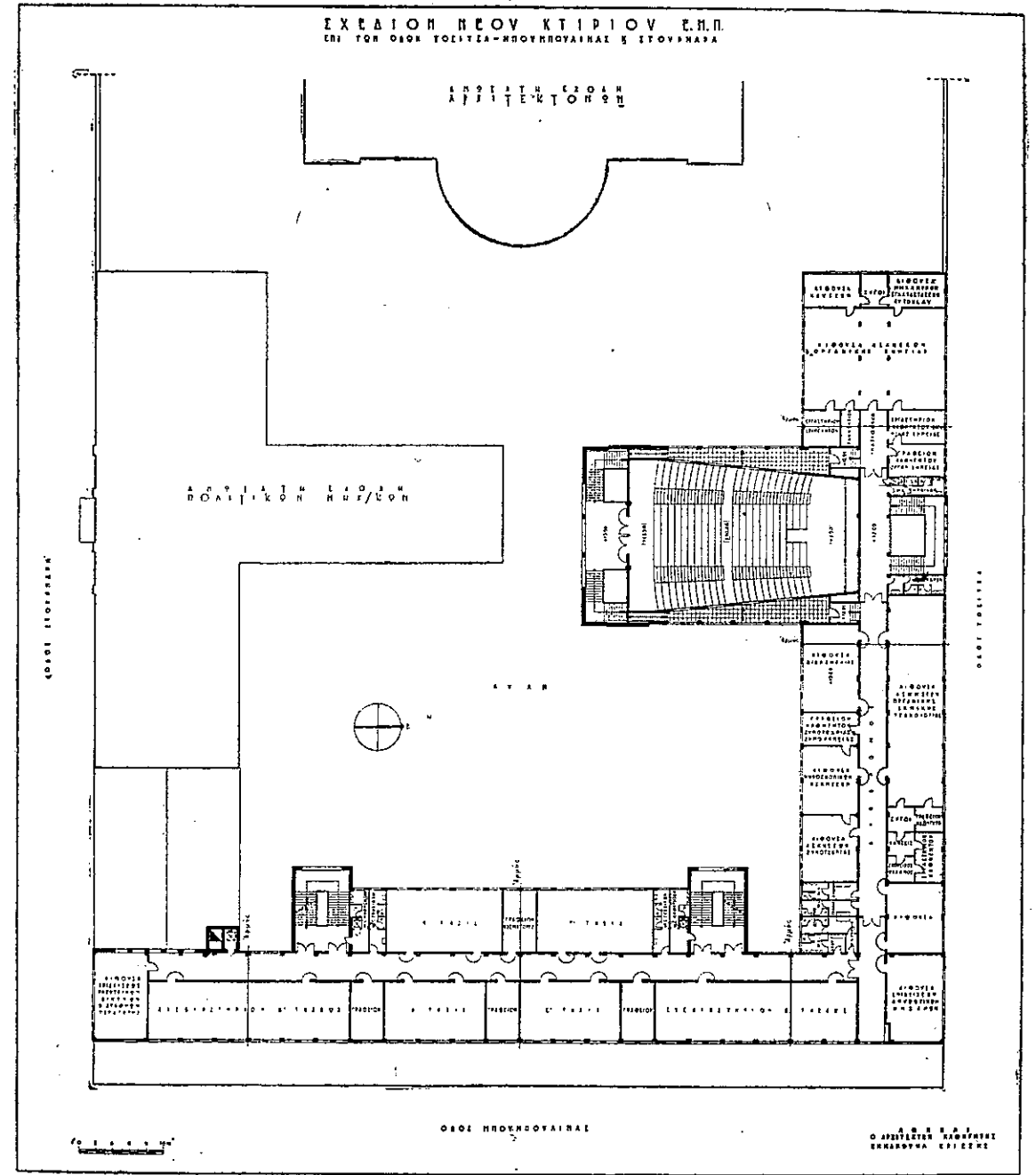
ΚΑΤΩΨΙΣ Γ'. ΟΡΟΦΟΥ
